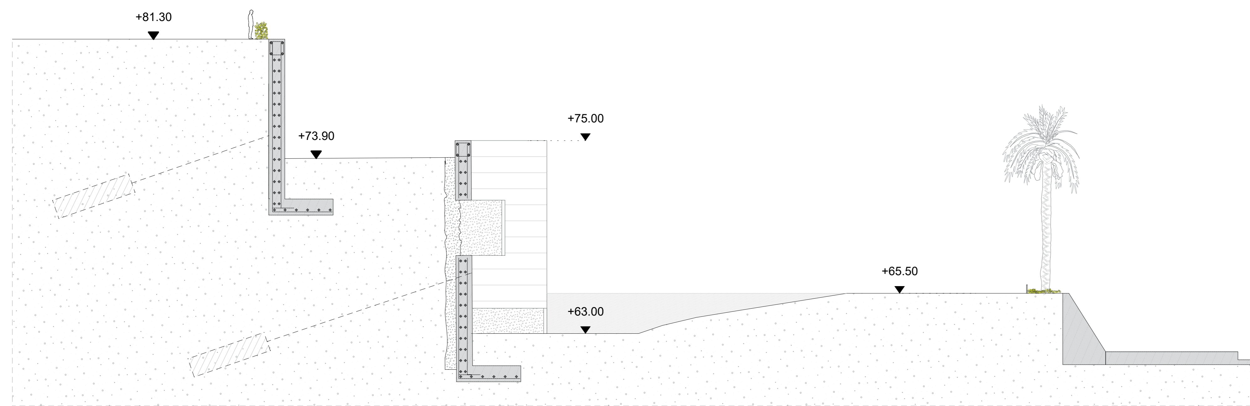
/ sección 1-1'
