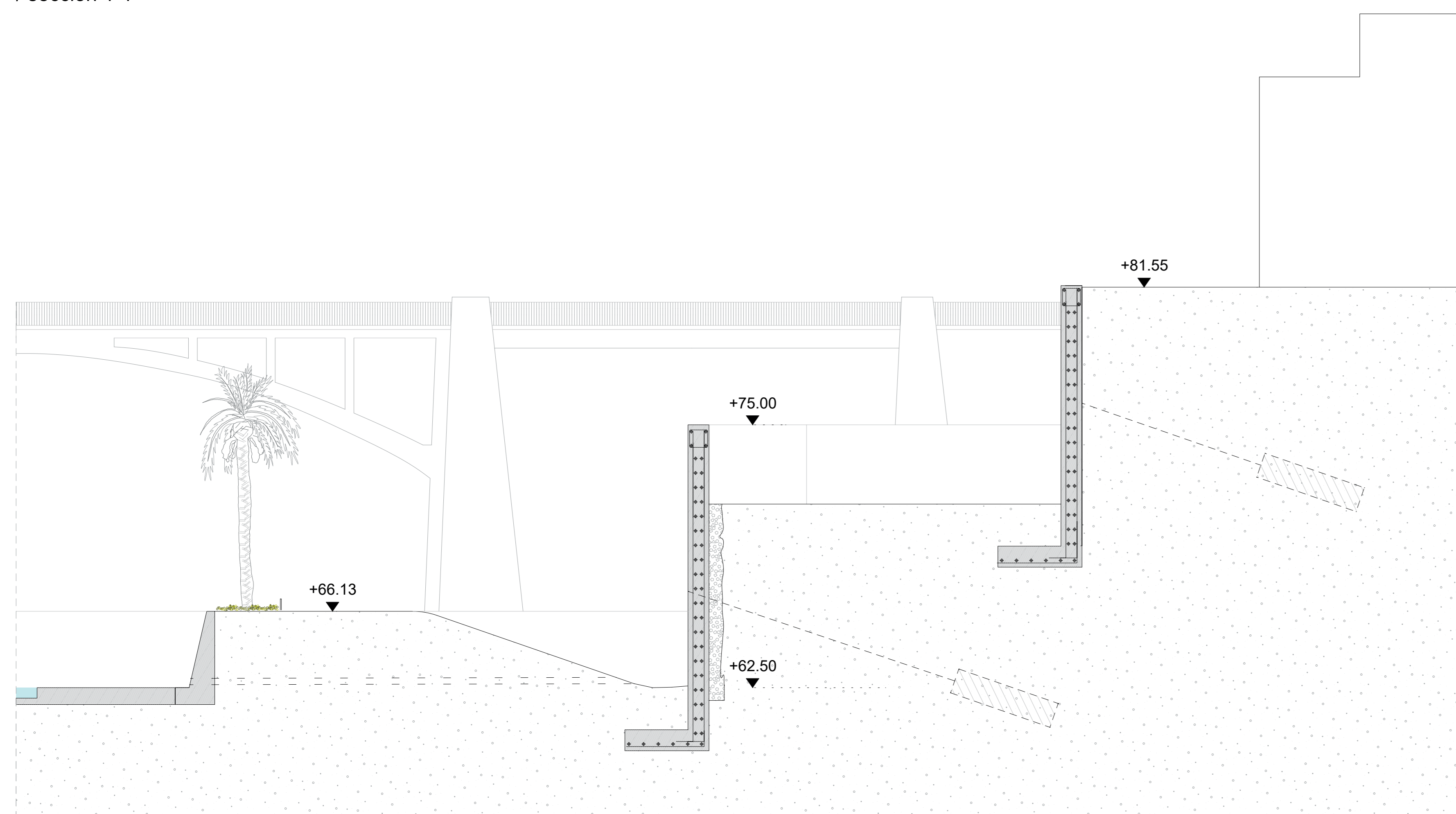
/ sección 1-1'
